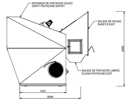
ALZADO FRONT
