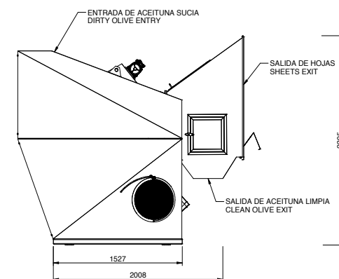
ALZADO FRONT
