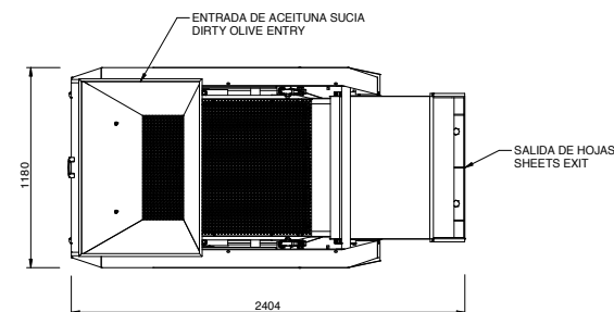
PLANTA TOP
