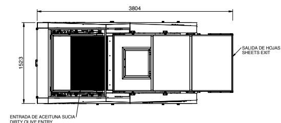
PLANTA TOP
